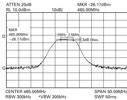
BPF中央频率 (出厂默认) C : 465MHz, C3 : 415MHz, C6 : 370MHz
