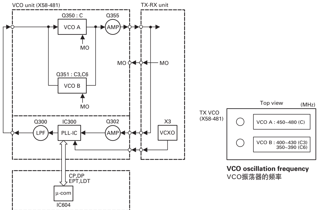
Fig. 6 Transmitter PLL / 图6 发射机PLL
